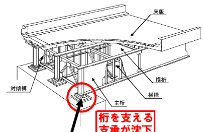
支承の損傷（沈下）
