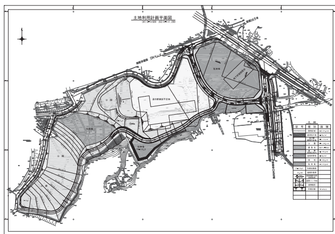
新道の駅建設事業土地利用計画平面図
