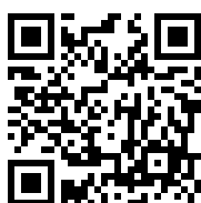
QRコード
