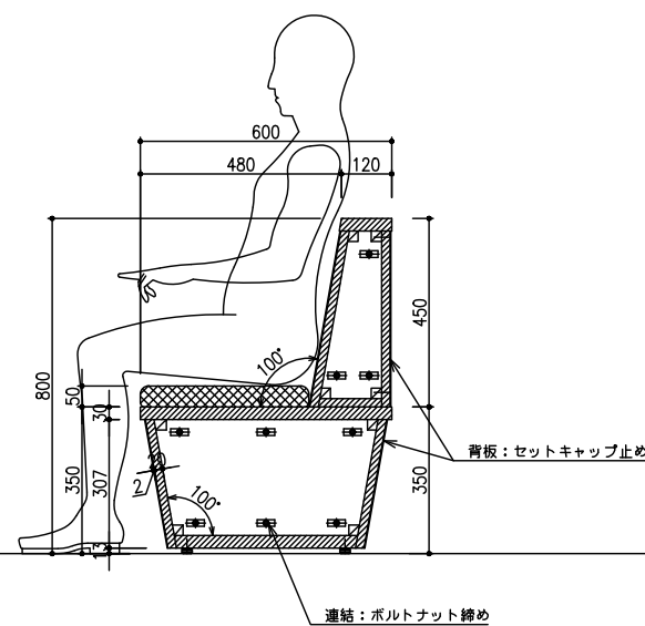
② 側断面図
