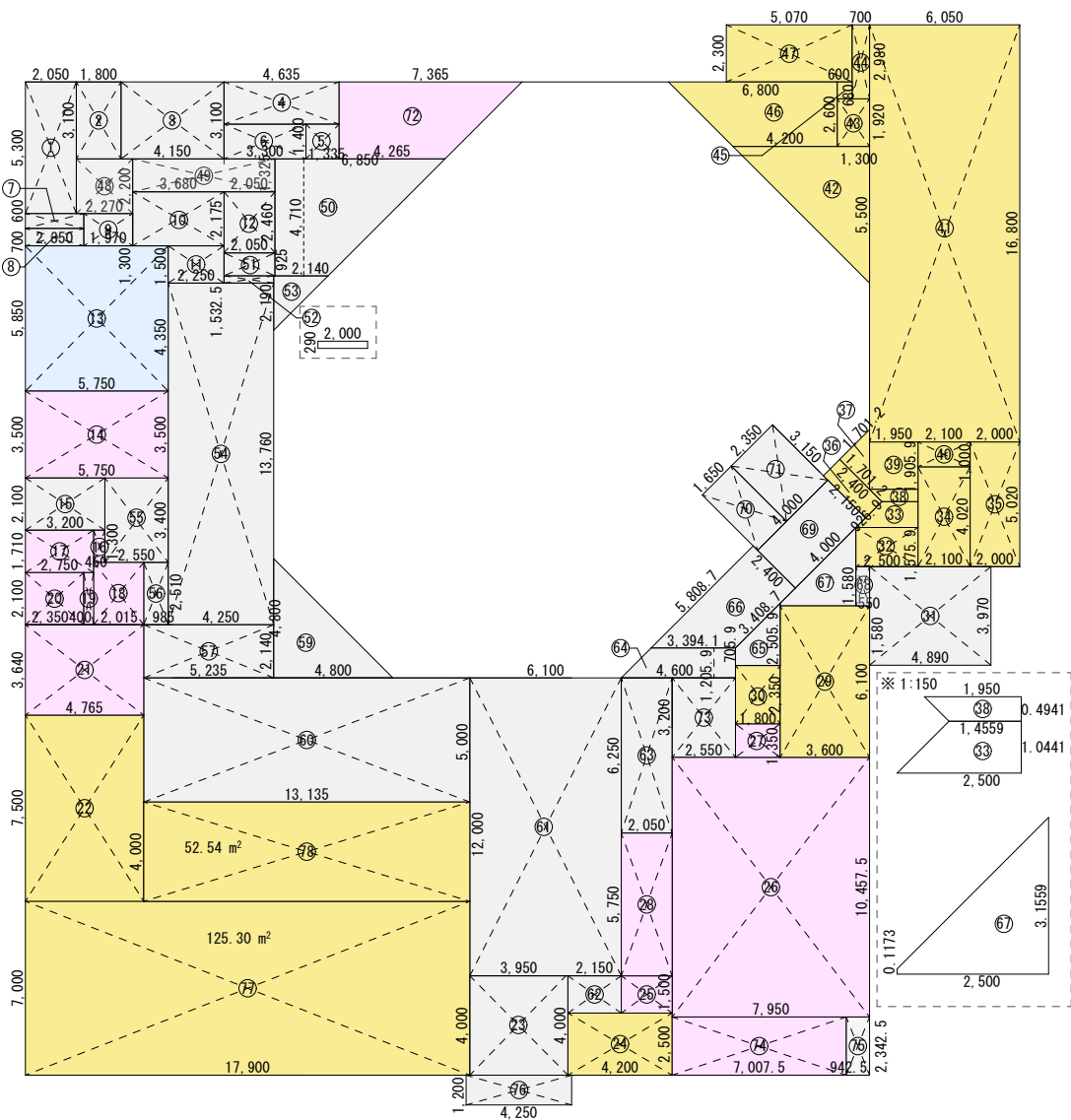
3階各室求積図 1:300
