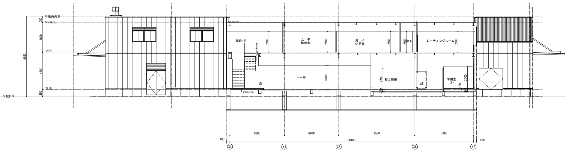
C-C断面図
