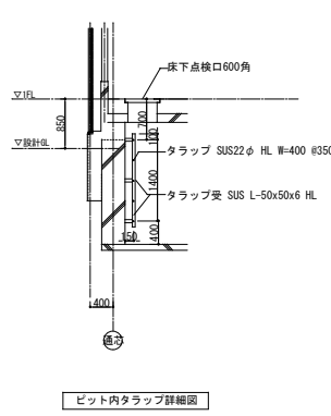
ビット内タラップ詳細図
