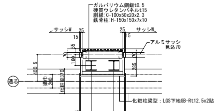
(A)部 詳細
