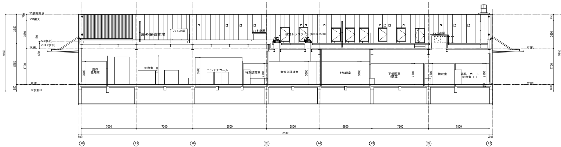
A'-A'断面図
