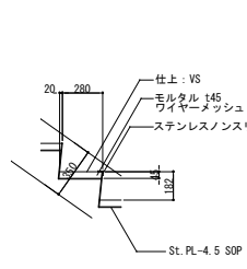
階段部詳細図
