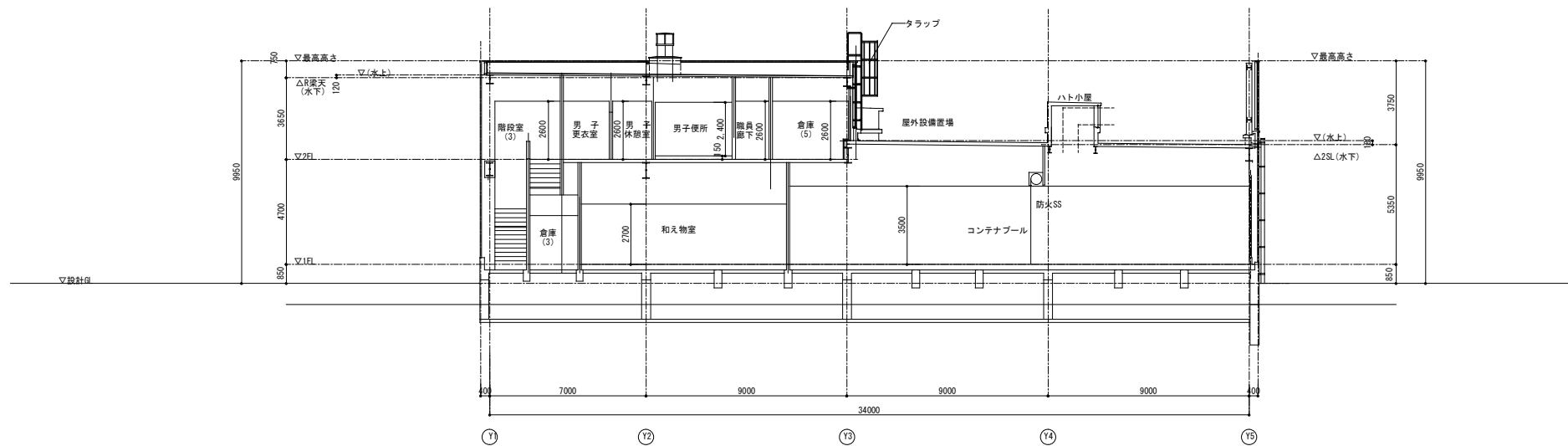
F-F断面図
