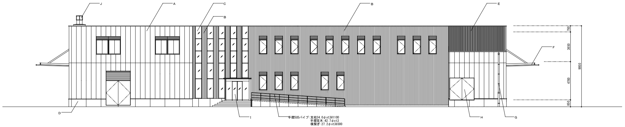
南立面図
