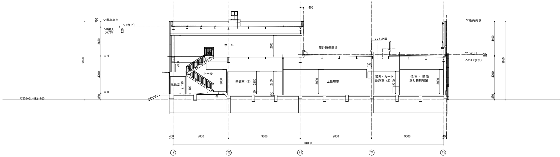
E-E断面図
