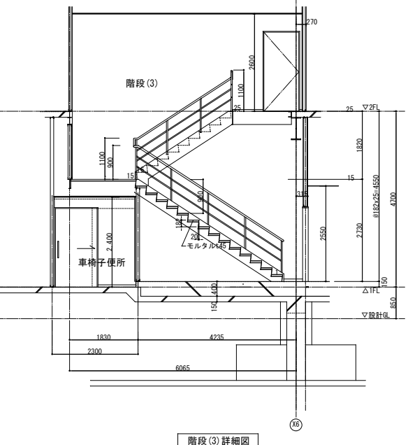
階段(3)詳細図
