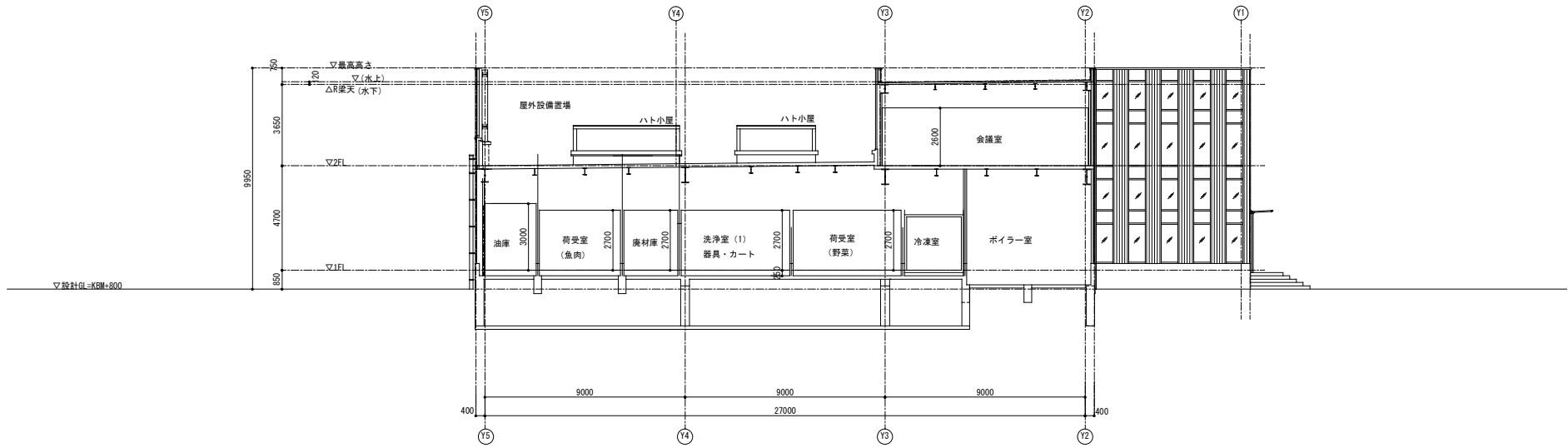
D-D断面図
