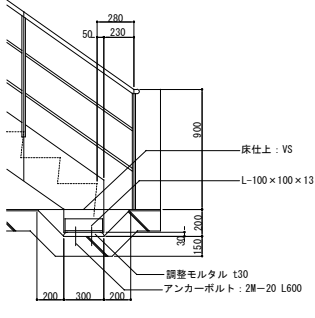
脚部詳細図
