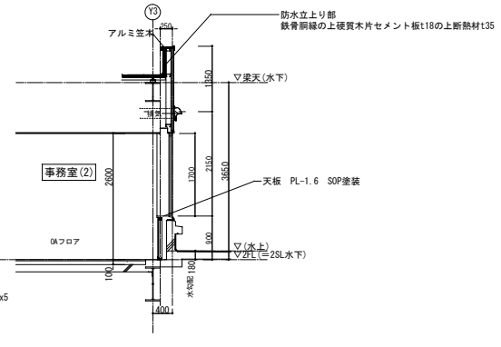
事務所(2) 断面詳細図
