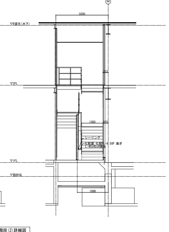
階段(2)詳細図
