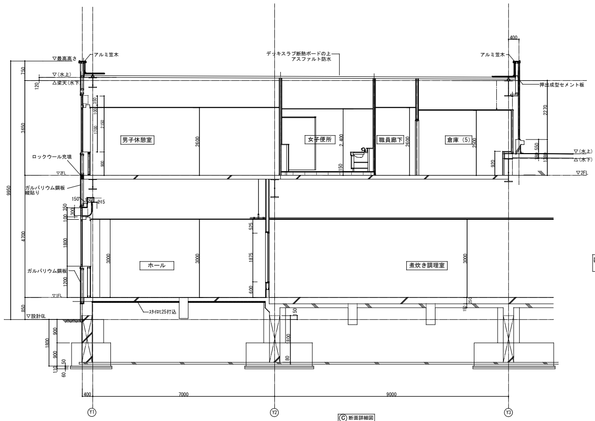
(C) 断面詳細図
