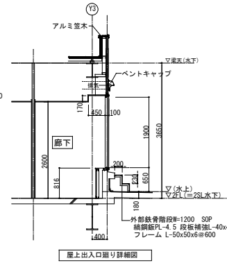
屋上出入口廻り詳細図
