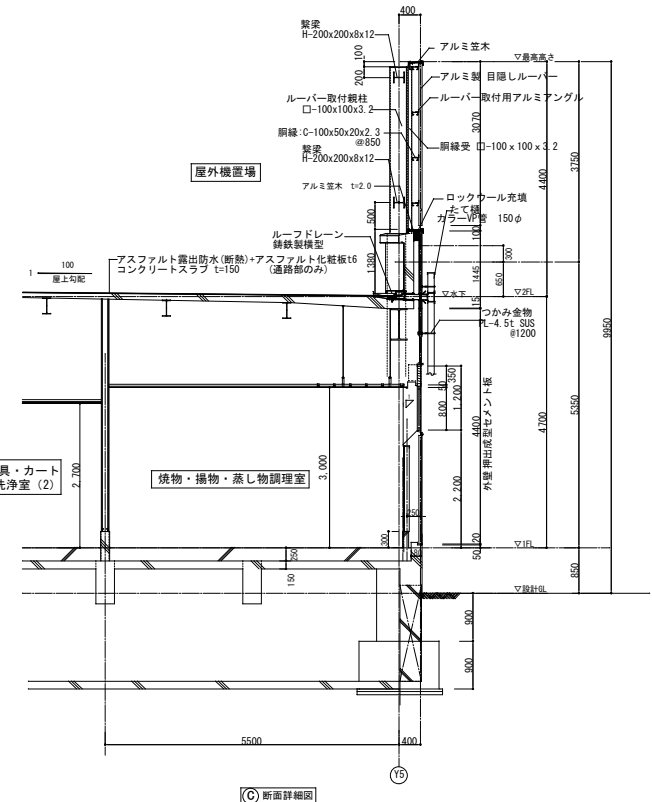
(C) 断面詳細図
