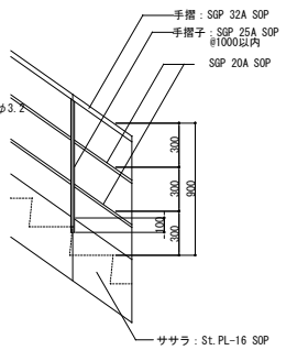
手摺詳細図
